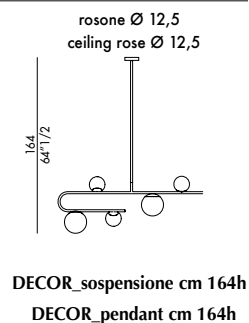
DECOR_3 sospensione DECOR_3 pendant
