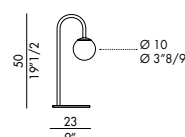
DECOR_1 tavolo DECOR_1 table
