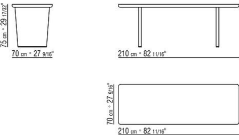
COD. 02F581 TABLE
