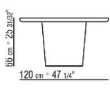
COD. 02F588 TABLE
